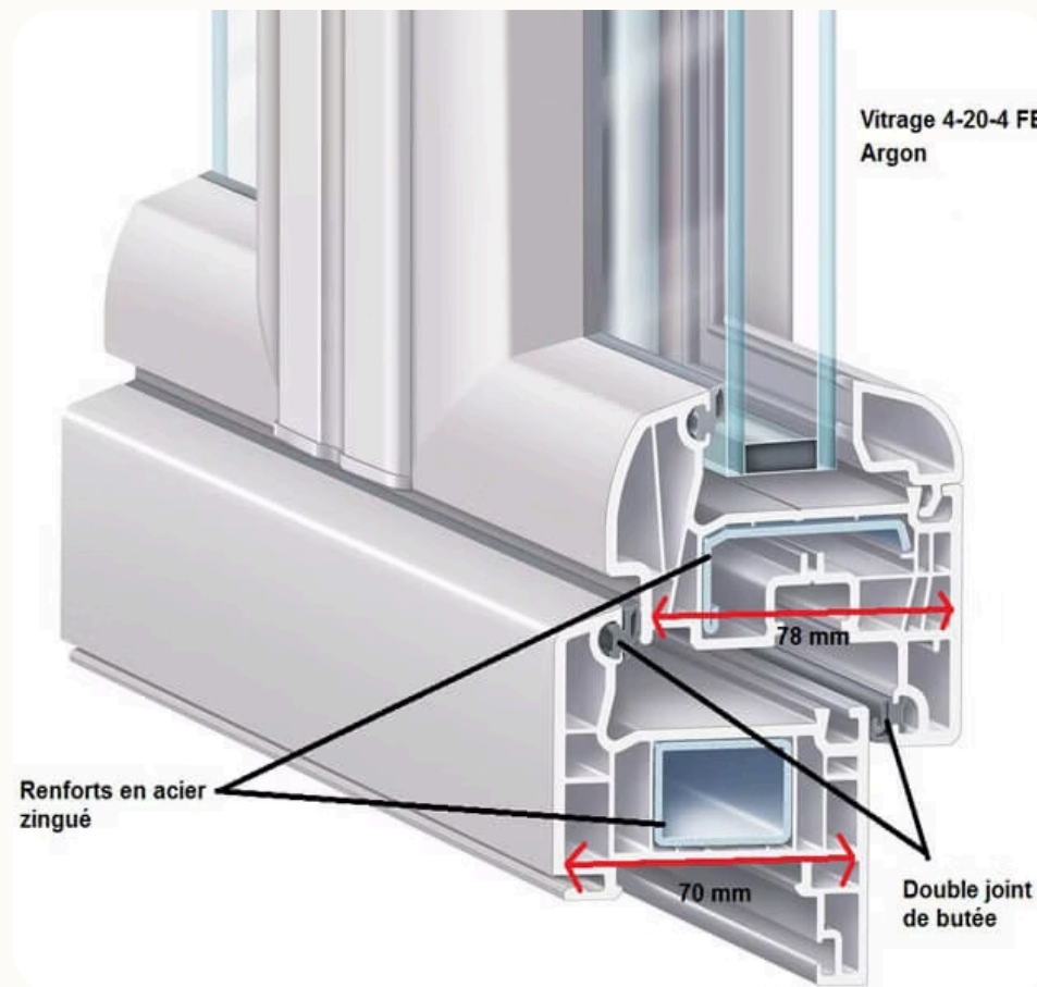
Coupe PVC
